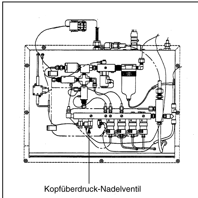
Abbildung 8-16. Einstellen des Kopfüberdruck-Nadelventils
